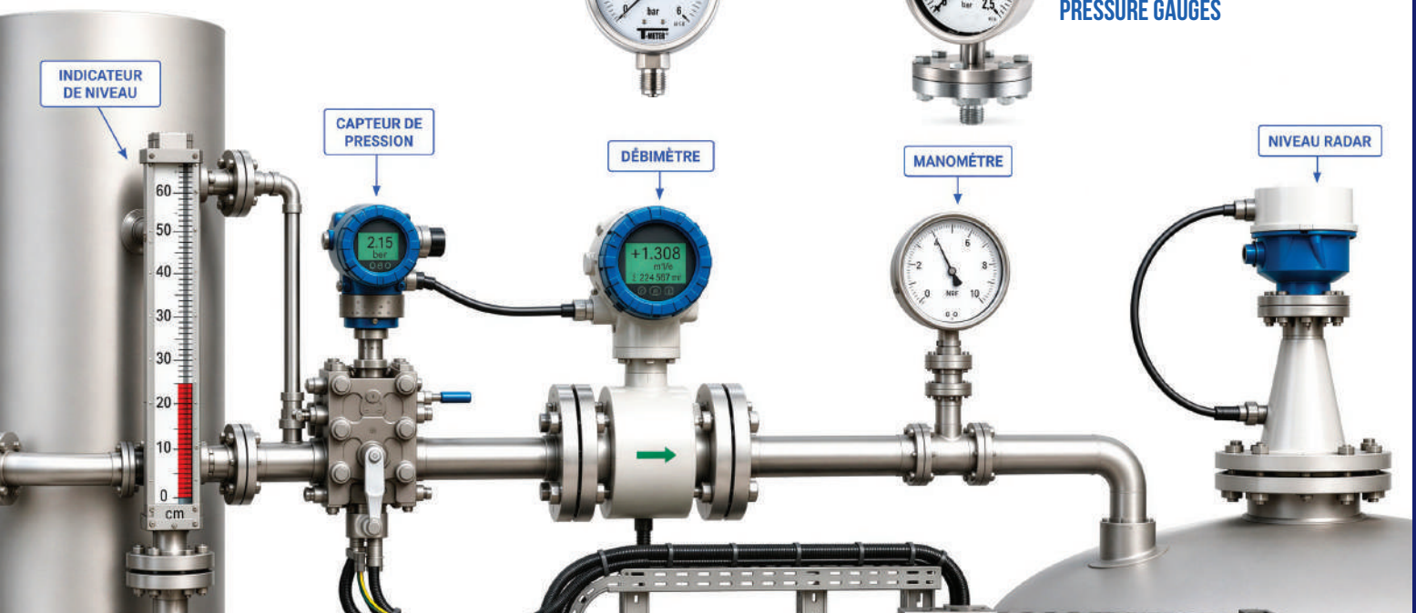
MANOMÈTRE
