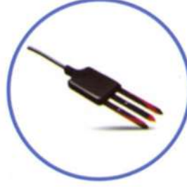
Sonde de mesure l'humidité, T° et EC du sol (USA & UK)
